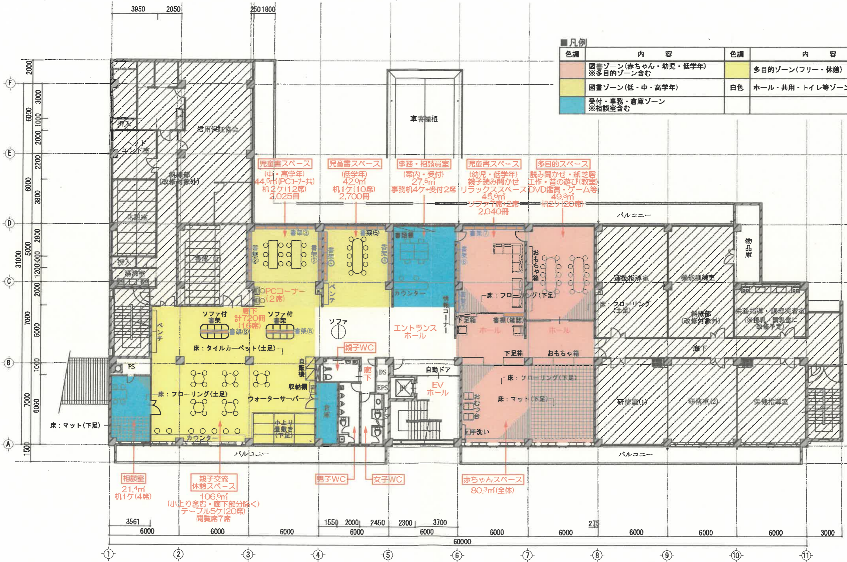
2F平面PLAN S=1/200
