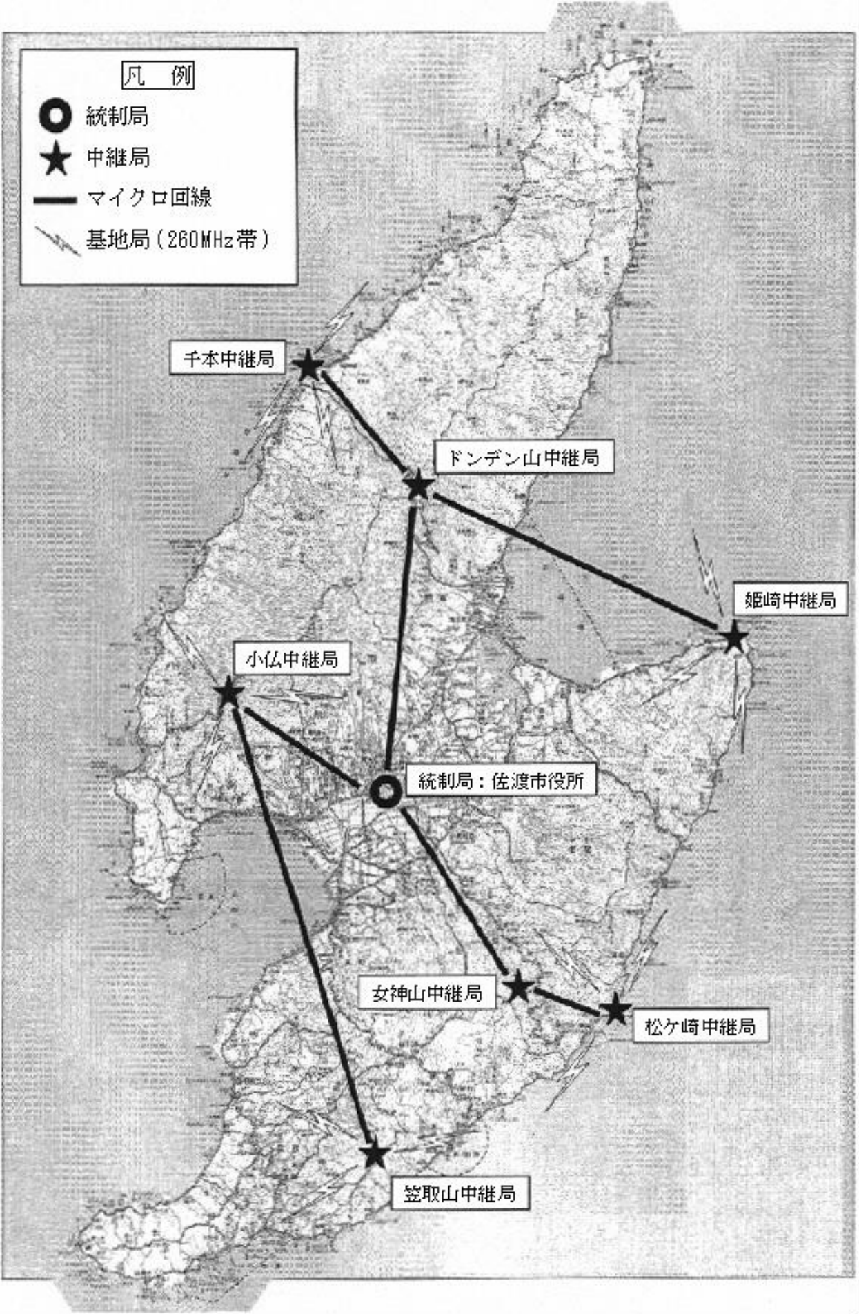
別表第1（第3条関係） 佐渡市デジタル防災行政無線システム構成図
