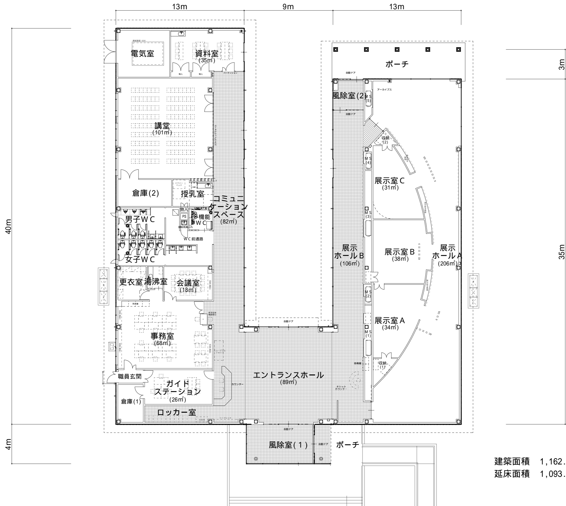
佐渡金銀山ガイド施設(仮称)建設(建築)工事 平面図
