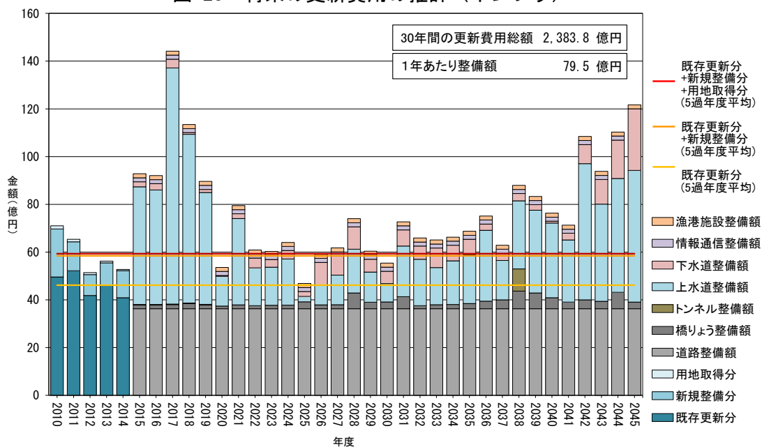
図 28 将来の更新費用の推計（インフラ）
