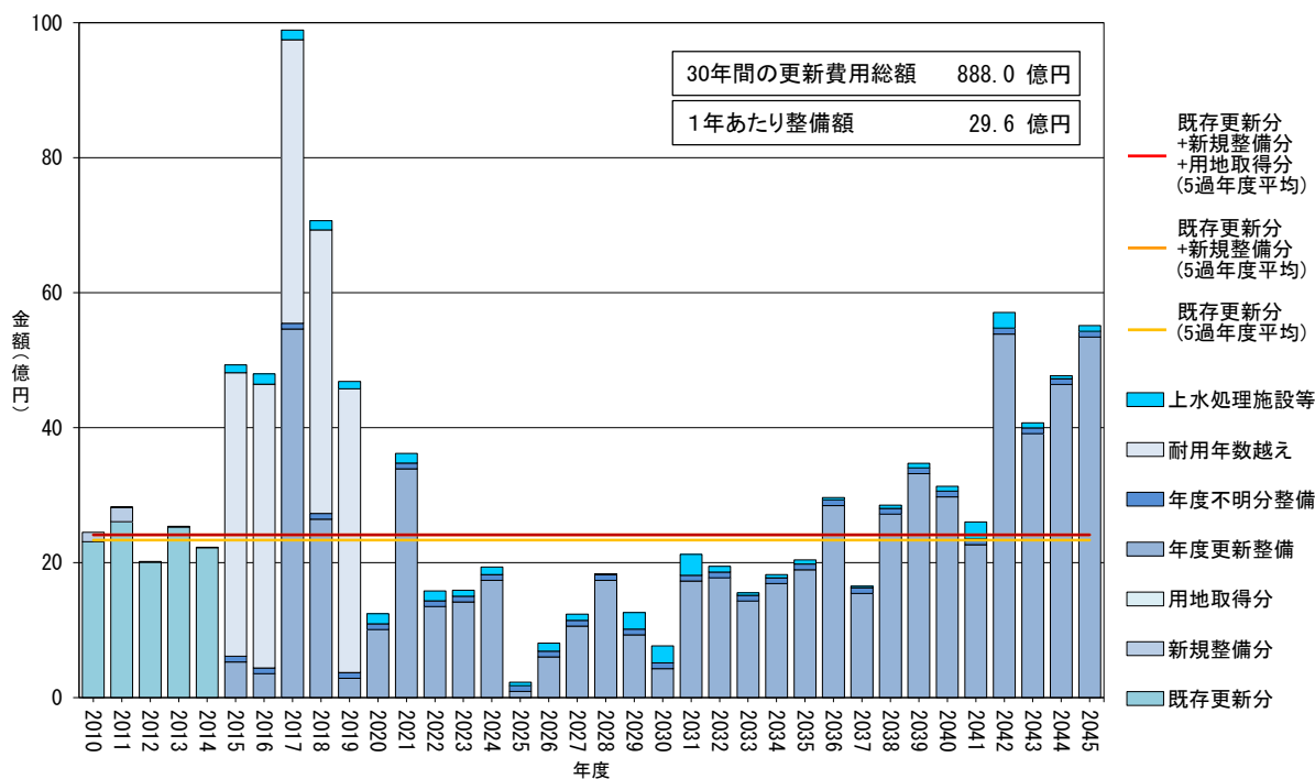
図 32 管径別・年度別延長による将来の更新費用の推計（上水道）
