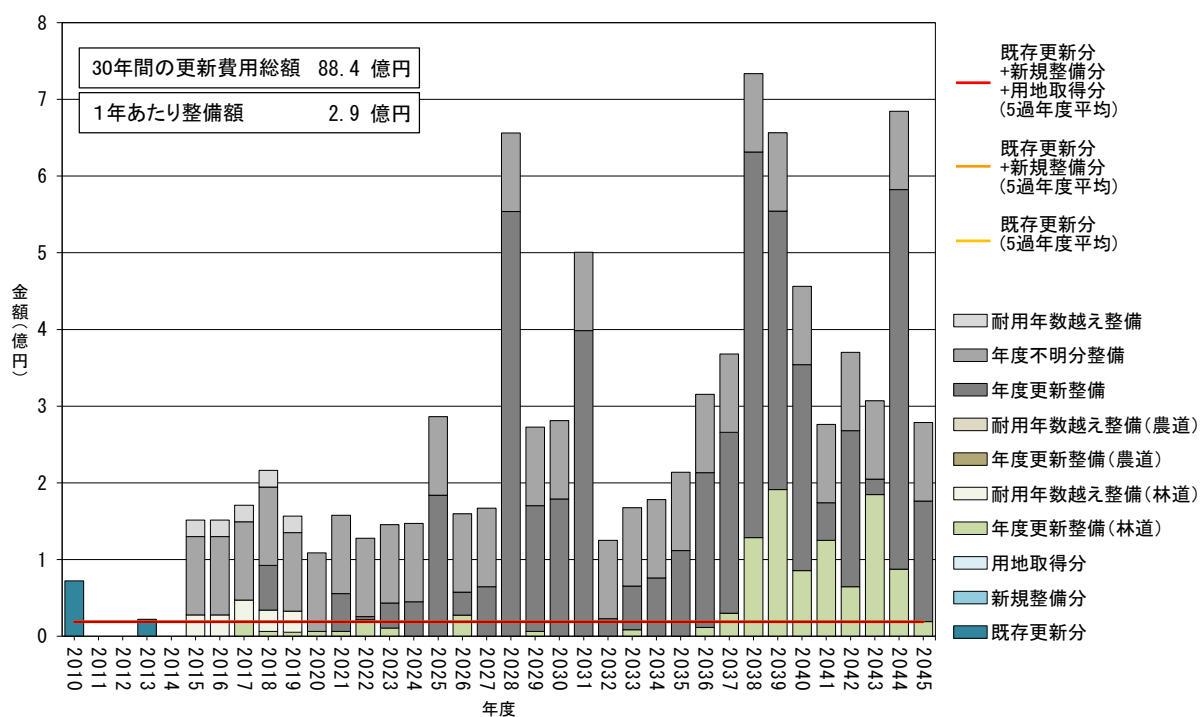
図 30 構造別面積による将来の更新費用の推計（橋梁）
