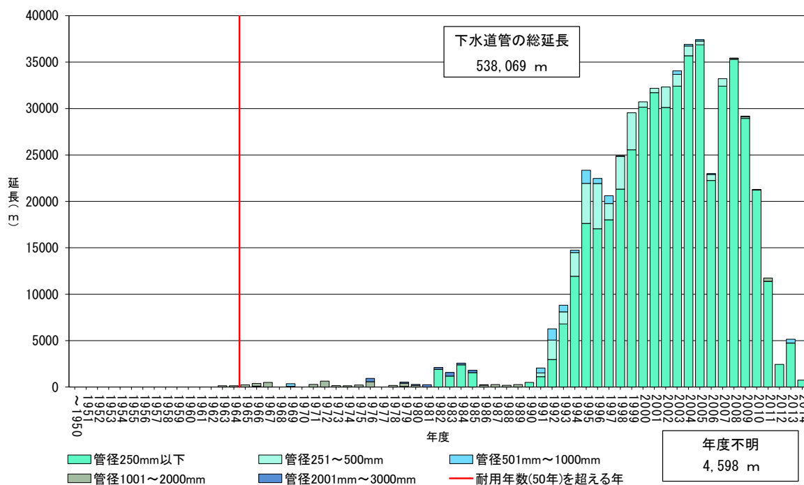
図 18 下水道（管渠）の年度別整備延長
