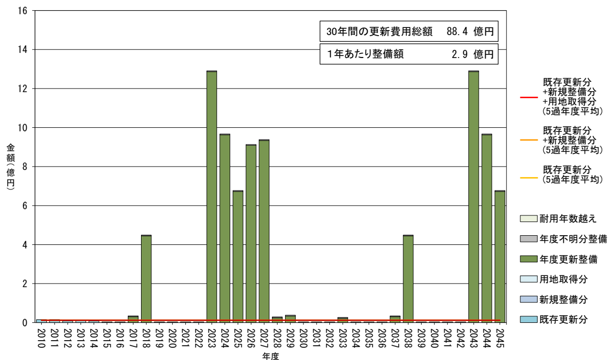
図 34 線種別・年度別延長による将来の更新費用の推計（情報通信ケーブル）
