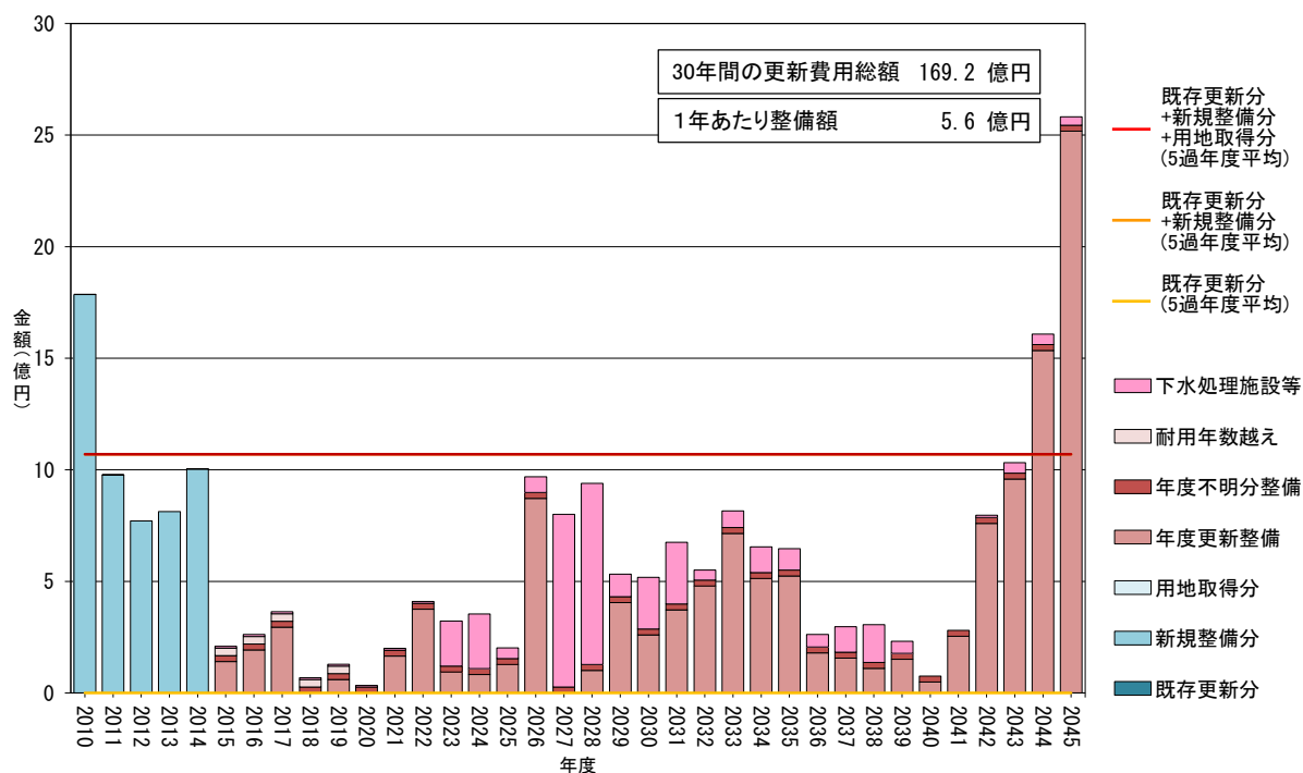
図 33 管径別・年度別延長による将来の更新費用の推計（下水道）
