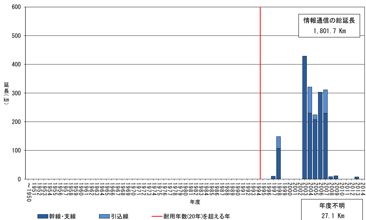
図 19 情報通信の年度別整備延長
