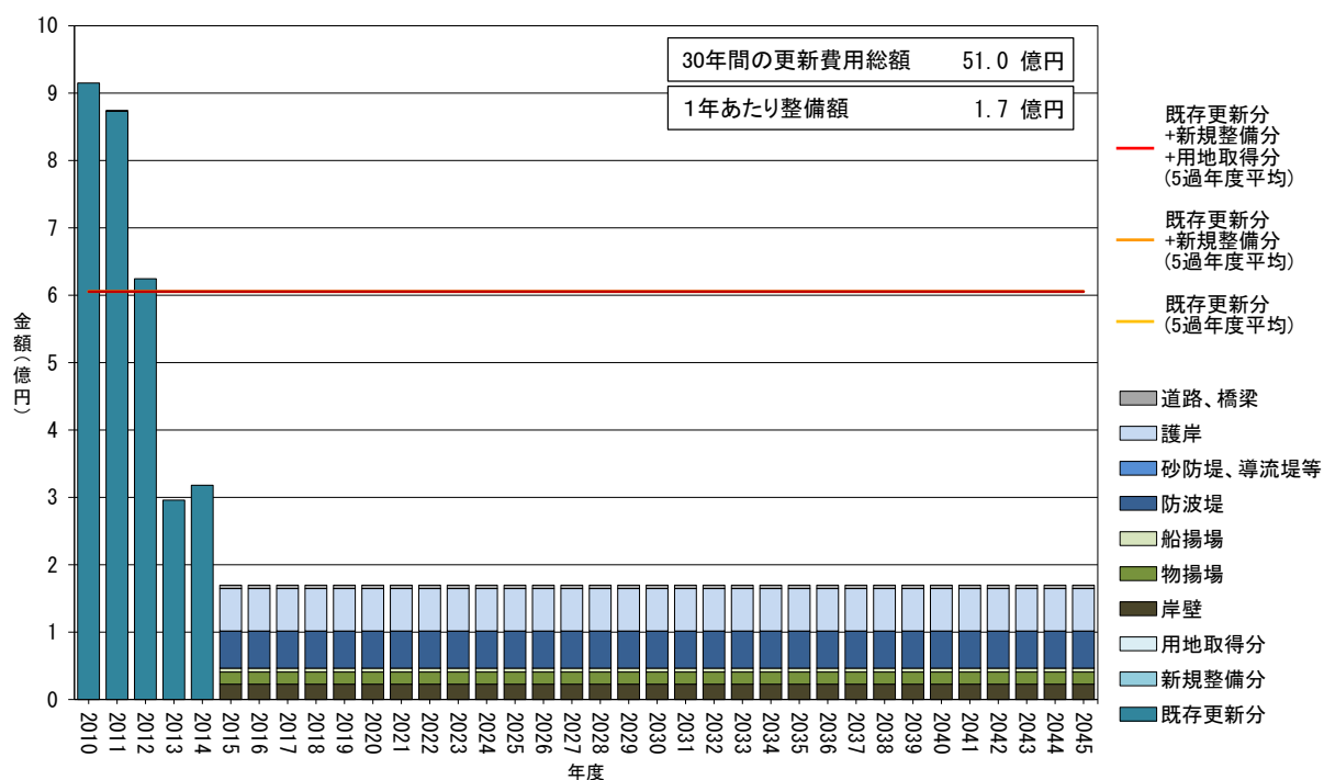
図 35 漁港機能保全計画による将来の更新費用の推計
