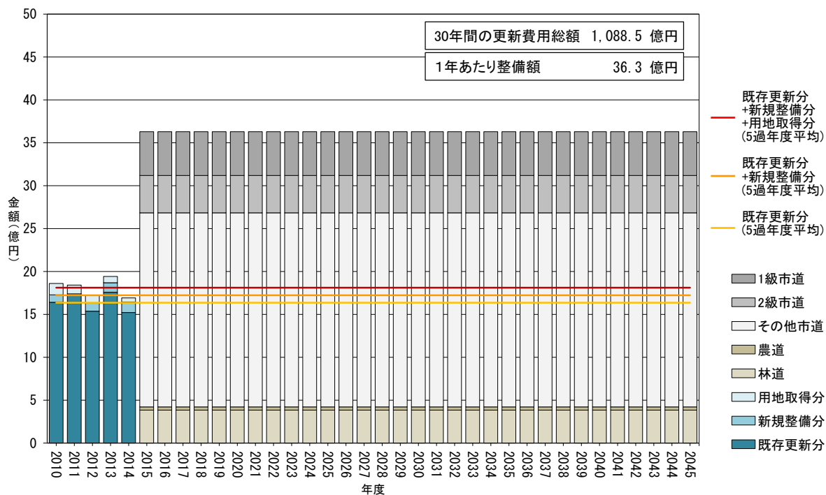
図 29 分類別面積による将来の更新費用の推計（道路）
