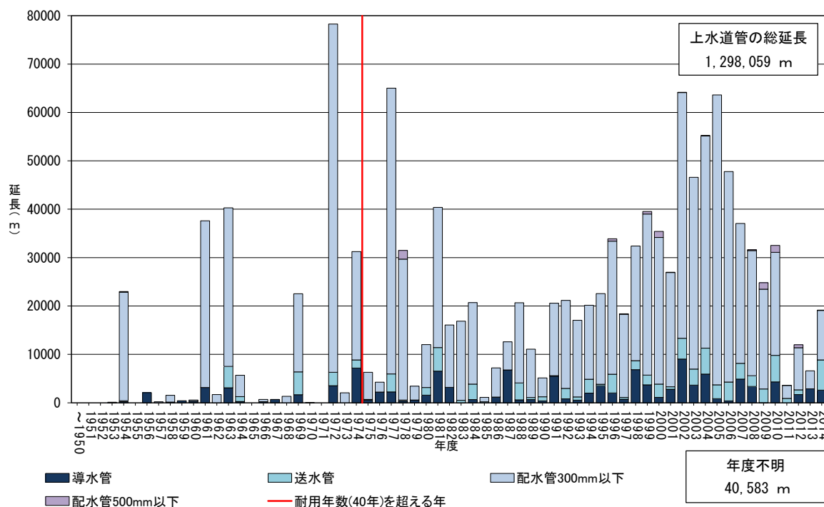
図 17 上水道（管渠）の年度別整備延長
