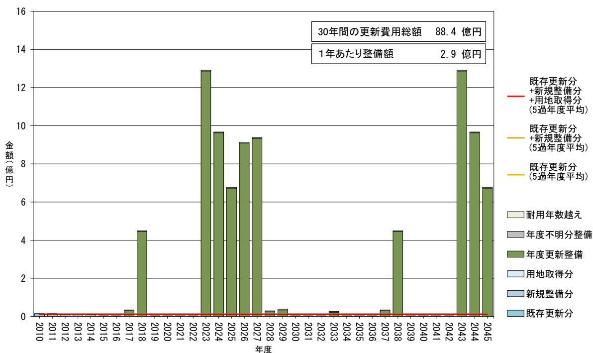
図 34 線種別・年度別延長による将来の更新費用の推計（情報通信ケーブル）
