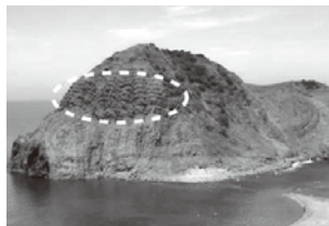
図1. 階段のように見える「節理」
