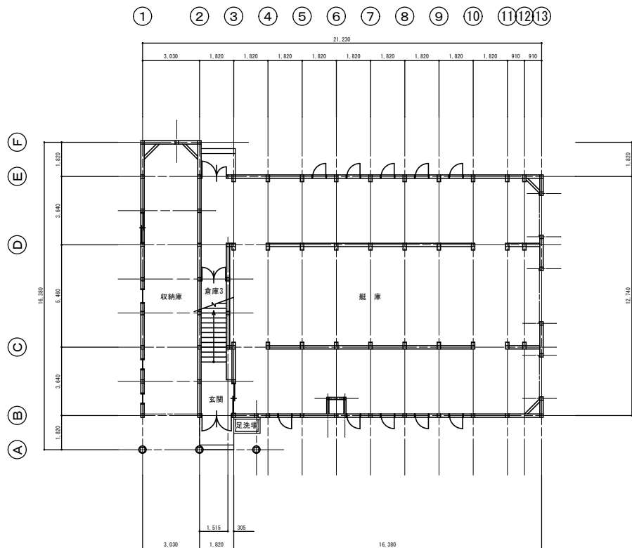
1階平面図
