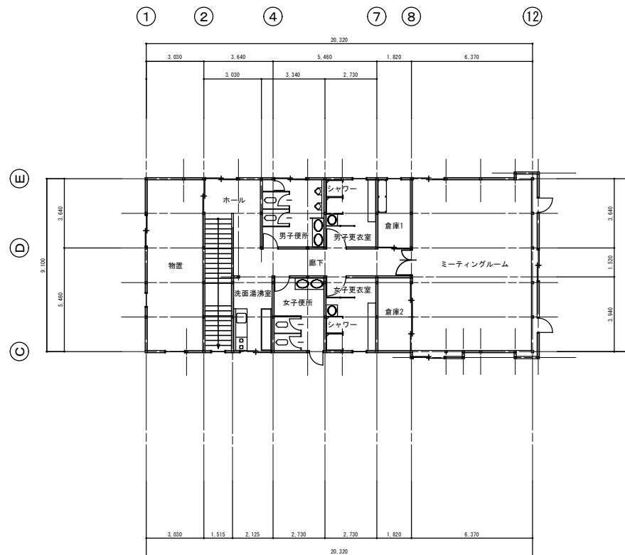
2階平面図
