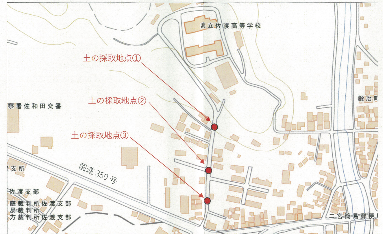
地質調査位置図
