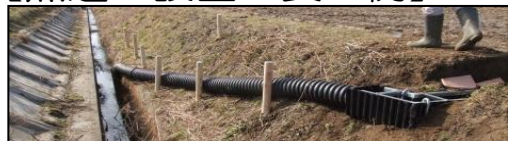
波付きの丸型水田魚道
