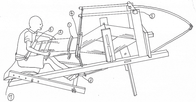
(図1)ネマリバタ 筆者作図
