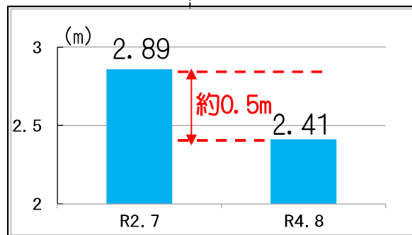
ピーク水位（島守水位観測所）
